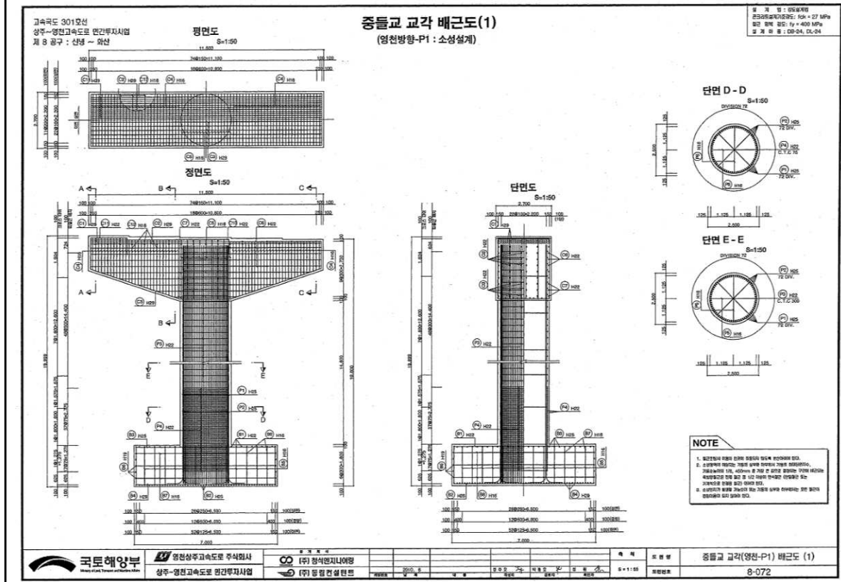
【그림 22.1.13】 교각 배근도
